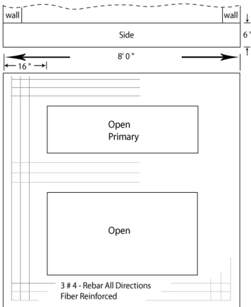
TV #3 - Footing Top (N.T.S)
