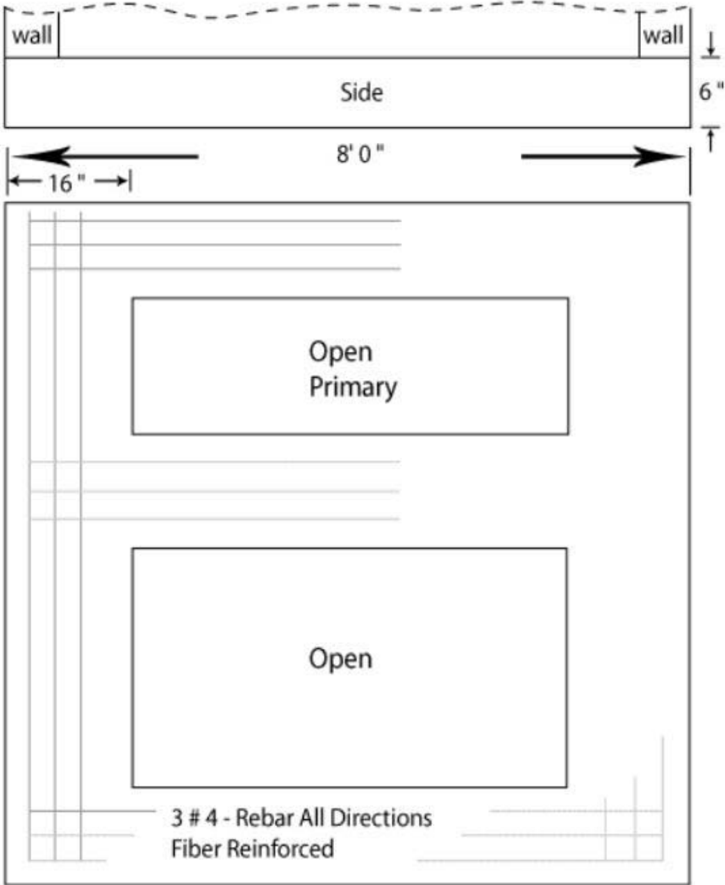
TV #3 - Footing Top (N.T.S)
